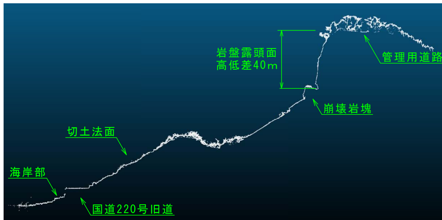
1-1断面
